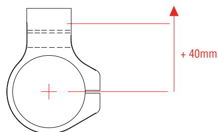
Bracciali manubrio con offset +40mm
