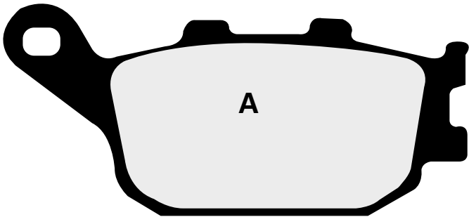
2P293 • A. 86,10 x 40 x 8,90mm / B. 86,10 x 40 x 8,9mm
