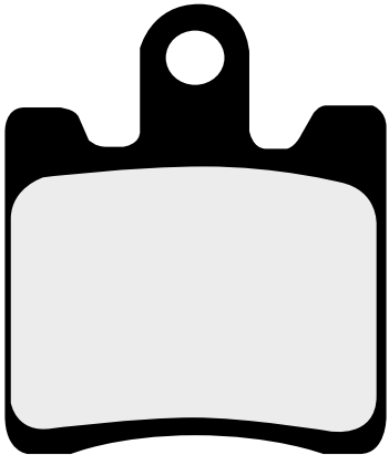
2P265 • 53,50 x 44,70 x 8,60mm
