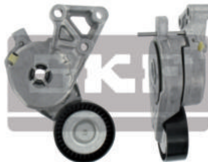
VKM 31011
